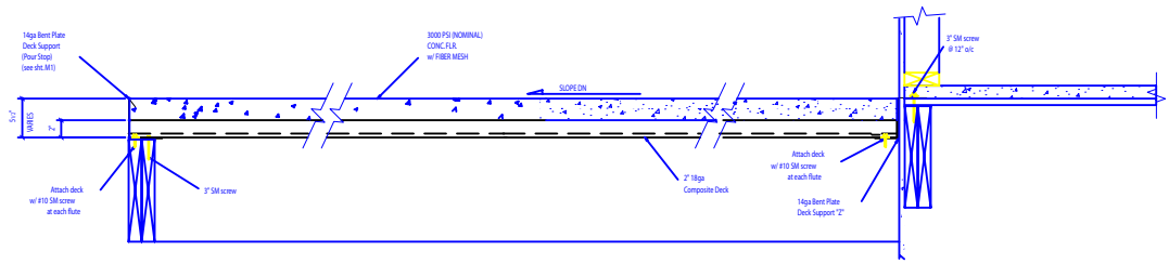
A E6 Section Thru Balcony
